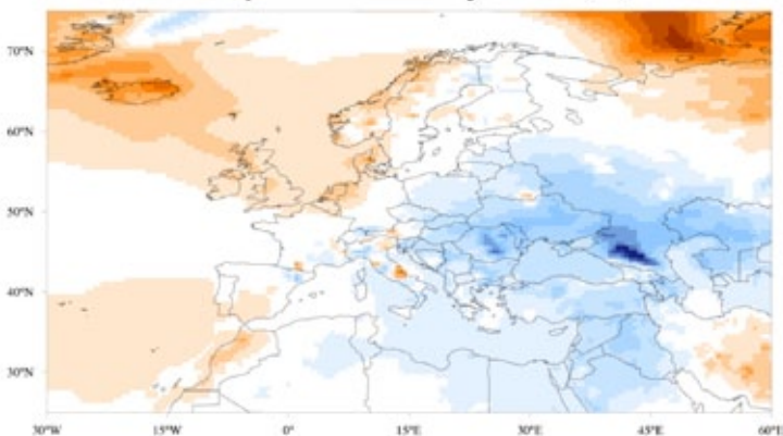
1979-1980 temperature anomaly at 2 m (°C)
