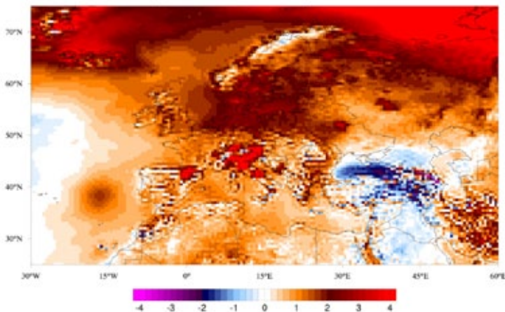
1979-1980 temperature anomaly at 2 m (°C)
